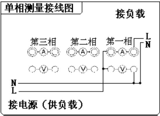
图 4-4 单相接线图
