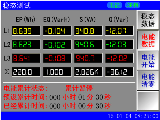
图 5-2 电能数据—停止状态
