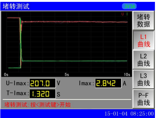
图 12-2 L1 曲线
