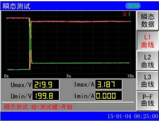
图 9-2 L1 曲线
