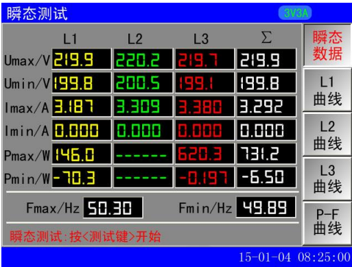
图 9-1 瞬态测试数据
