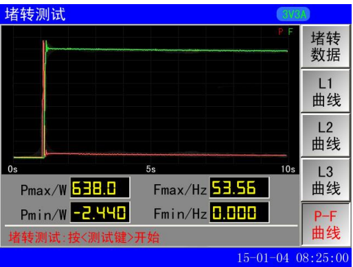
图 12-3 P-F 曲线
