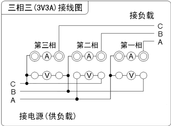
图 4-7 3V3A 接线图
