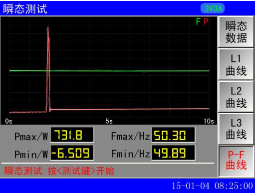
图 9-3 P-F 曲线
